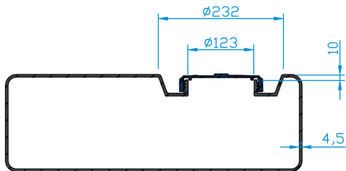
ŘEZ A-A
