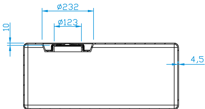
ŘEZ A-A
