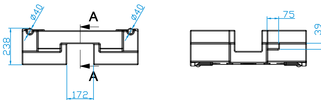
ŘEZ A-A M 1:8
