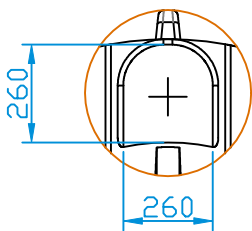
Detail odtoku (1:20)
