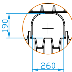
Detail nátoku (1:20)
